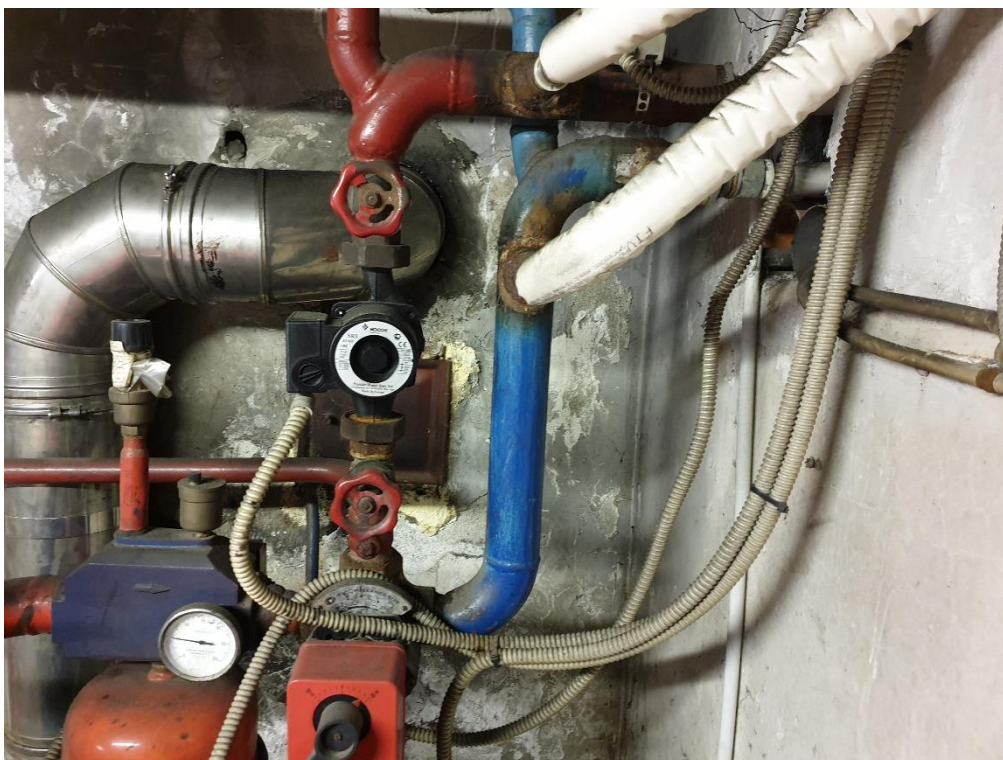
Foto 3 – Circolatori circuito anticondensa e circuito riscaldamento Palazzo Comunale
